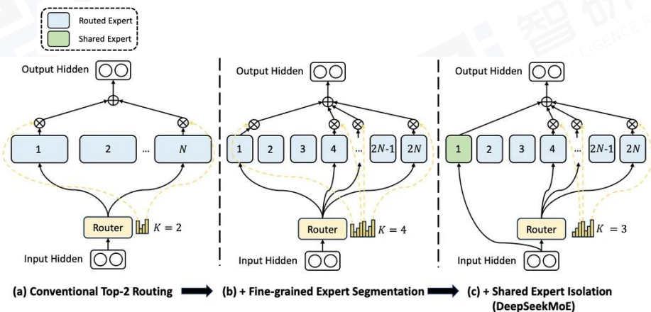
DeepSeek MoE与传统MoE的区别
