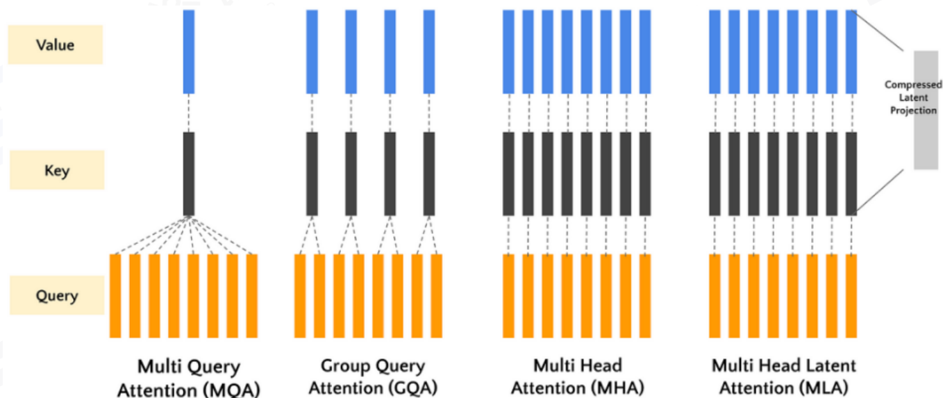
MHA、MQA、GQA 与 MLA
